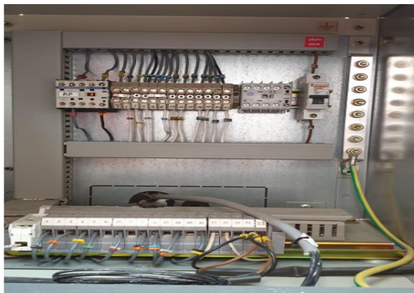
איור ג'- תא פיקוד טיפוסי לכל התאים
